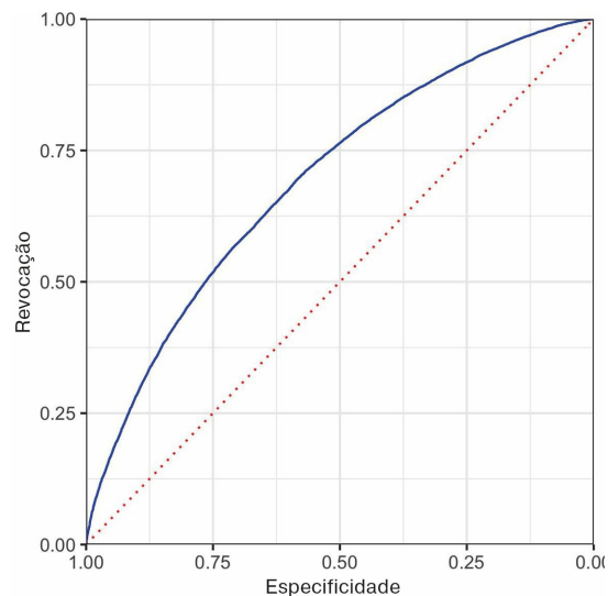
Figura 5-6. Curva ROC para os dados de empréstimo
