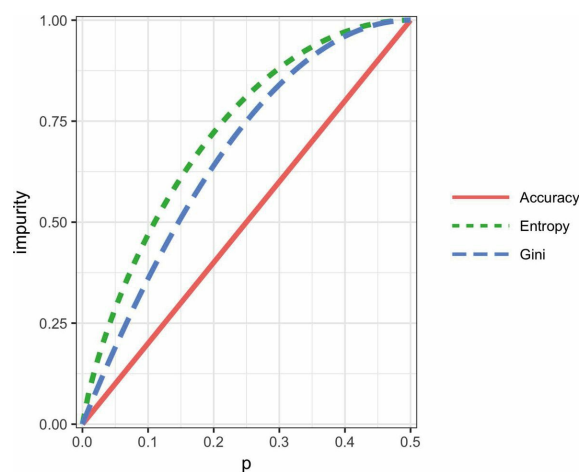
Figura 6-5. Medidas de impureza de Gini e entropia
