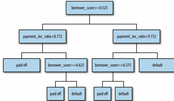
Figura 6-3. As regras para um modelo de árvore simples ajustado aos dados de empréstimo
