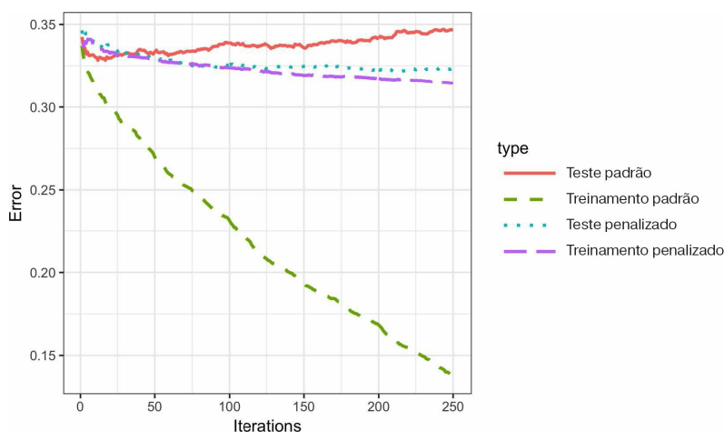
Figura 6-10. A taxa de erro do XGBoost padrão contra a versão penalizada de XGBoost
