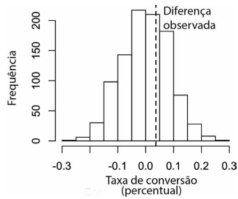
Figura 3-5. Distribuição de frequências para a diferença entre taxas de conversão entre as páginas A e B
