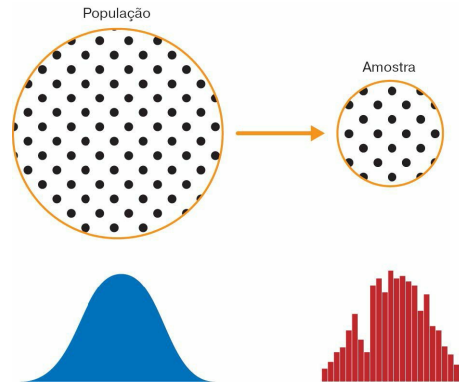
Figura 2-1. População versus amostra
