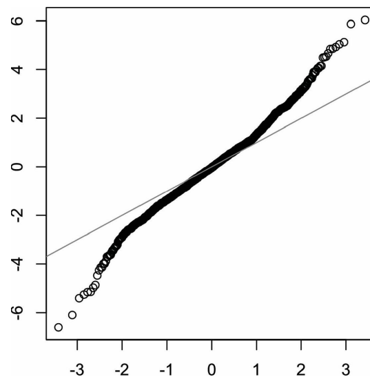
Figura 2-12. Gráfico QQ dos retornos da NFLX
