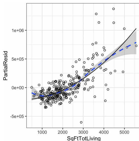
Figura 4-12. Uma regressão spline ajustada para a variável SqFtTotLiving (linha sólida) comparada com uma suavização (linha tracejada)
