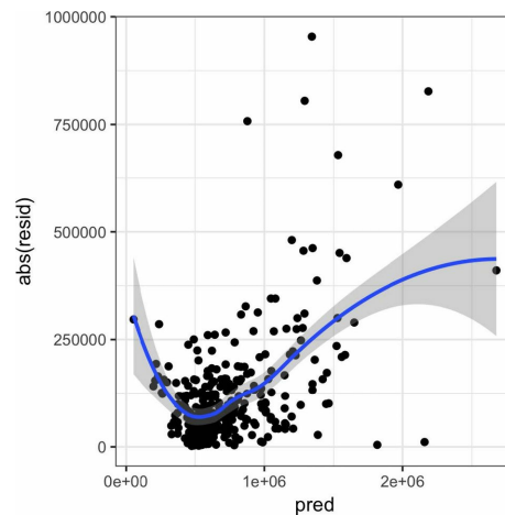
Figura 4-7. Um gráfico do valor absoluto dos resíduos versus os valores previstos
