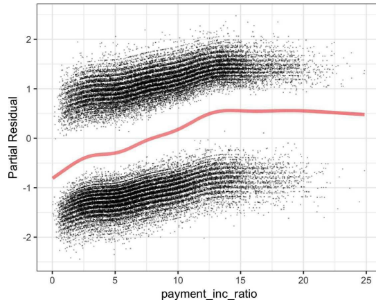
Figura 5-4. Resíduos parciais da regressão logística
