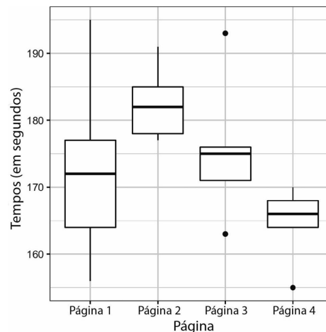
Figura 3-6. Boxplots dos quatro grupos mostrando diferenças consideráveis entre si
