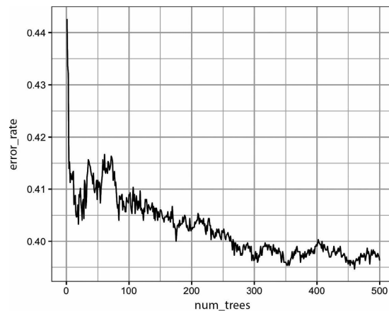
Figura 6-6. A melhora em precisão da floresta aleatória com a adição de mais árvores
