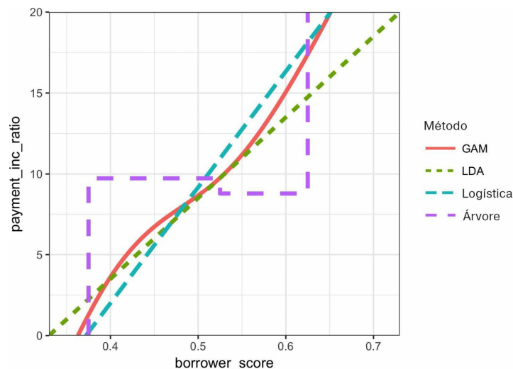
Figura 5-8. Comparação entre as regras de classificação para quatro métodos diferentes
