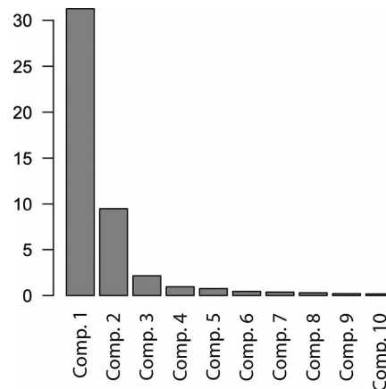
Figura 7-12. Um screeplot para um PCA das principais ações do S&P 500 incluindo GOOGL e AMZN
