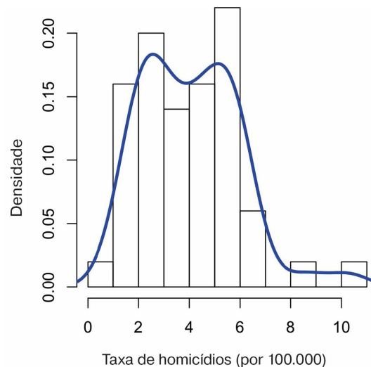
Figura 1-4. Densidade das taxas de homicídio estaduais
