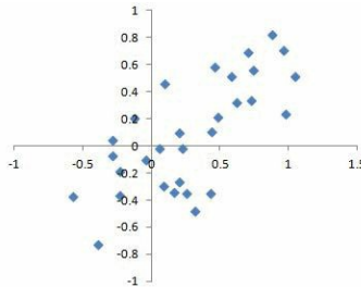
Figura 2-3. Gráfico de dispersão de tiros de uma arma com alvo enviesado
