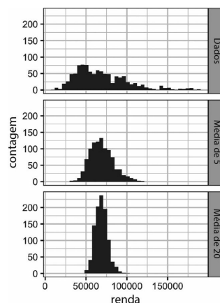
Figura 2-6. Histograma de rendimentos anuais de 1.000 candidatos a empréstimo (topo), então 1.000 médias de n = 5 candidatos (meio), e n = 20
