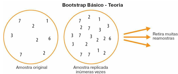
Figura 2-7. A ideia do bootstrap
