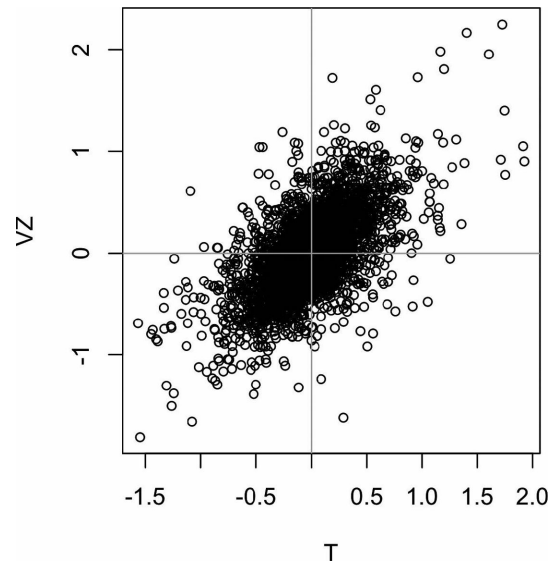
Figura 1-7. Gráfico de dispersão entre os retornos das empresas ATT e Verizon
