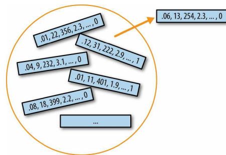
Figura 2-8. Amostragem bootstrap multivariada
