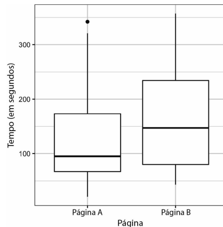
Figura 3-3. Tempos de sessão para as páginas web A e B
