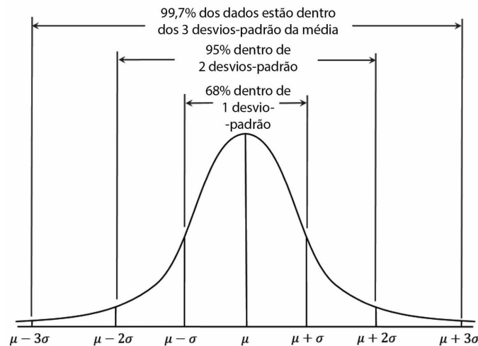
Figura 2-10. Curva normal
