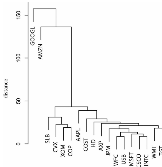
Figura 7-7. Um dendrograma de ações
