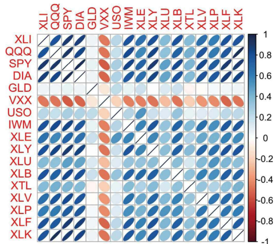
Figura 1-6. Correlação entre retornos de ETF
